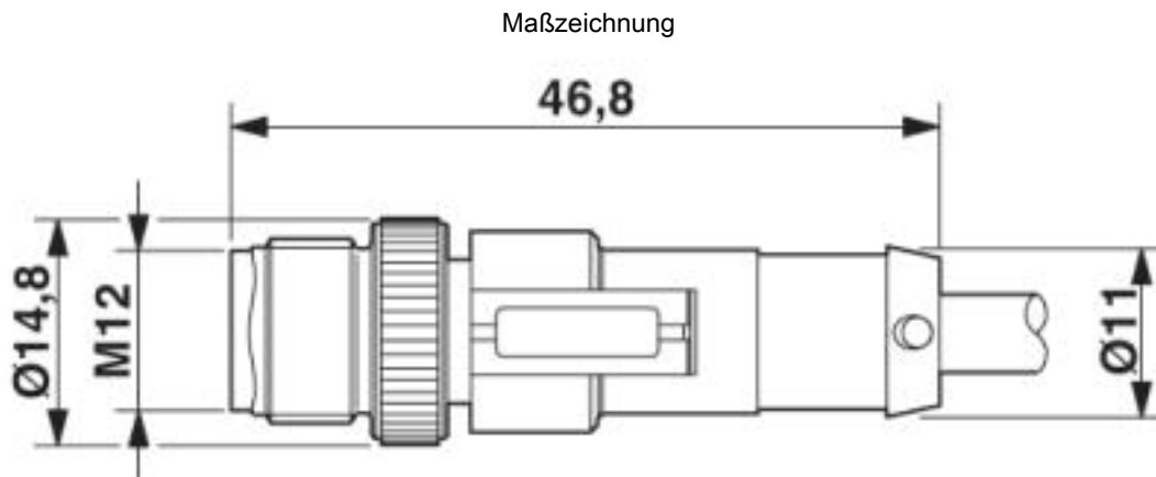
Stecker M12 x 1, gerade, geschirmt
