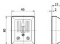
Katalog- Maßzeichnung
